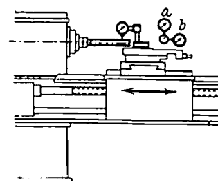
Fig. 55. Spindle
