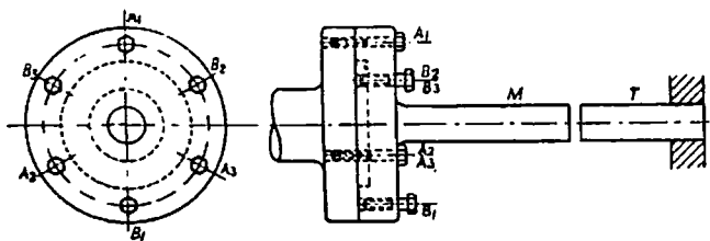
Fig. 51. Double Mandrel Test
